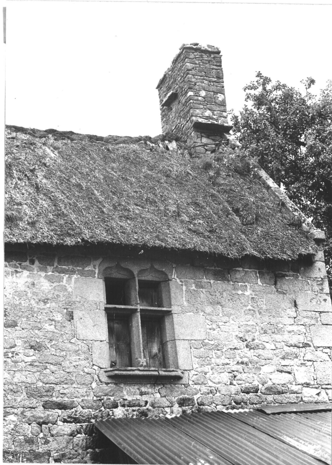
44/11 - Croisée du second niveau à encadrement à cavet, linteau à double accolade, meneau élégant et orné à la base, appui mouluré.
