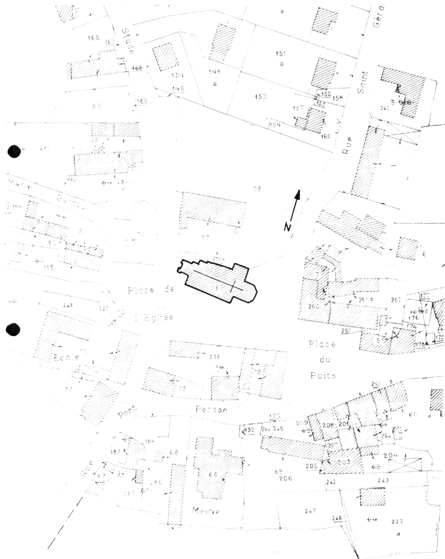
Pl. I Plan de situation. Extrait cadastral 1980, section AB, échelle 1/1000 e .
