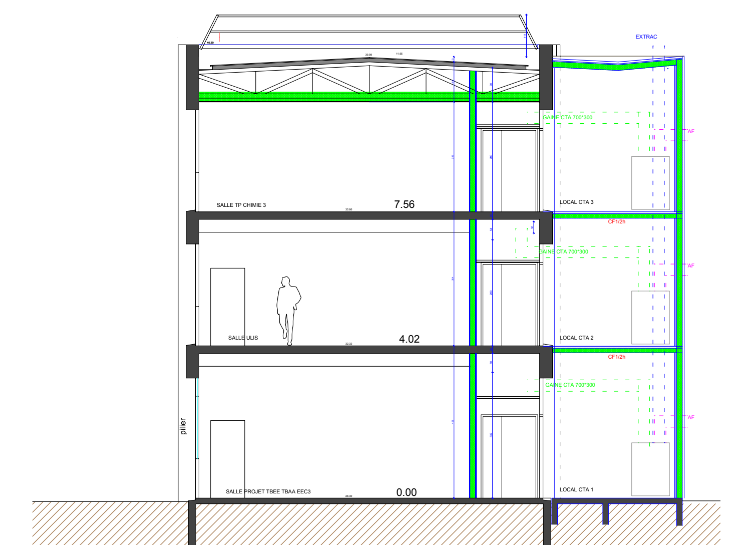
COUPE BB
