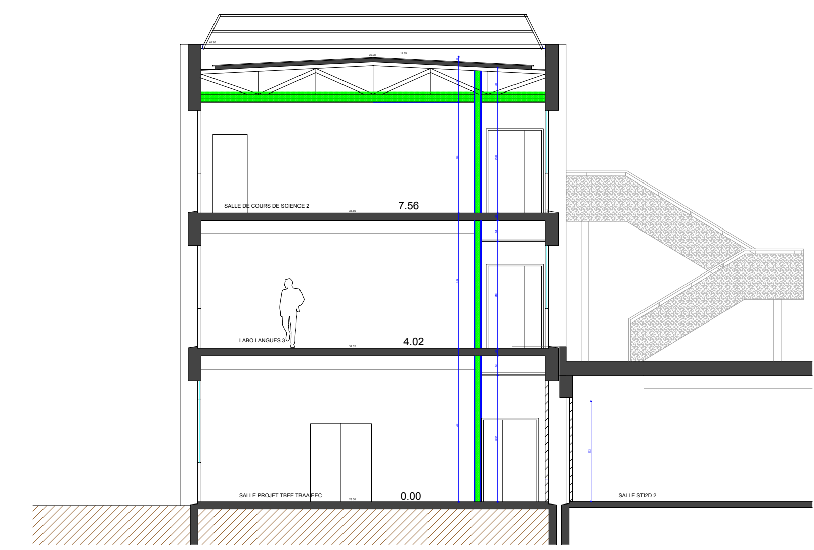
COUPE AA
