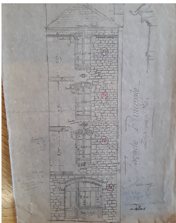
Plan et état actuel de la façade au 4 rue Lobineau. Source : Archives de Rennes, 769 W 25, Permis de construire.
