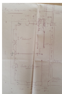
Plan du rez-de-chaussée surélevé du 24 rue Villeneuve
