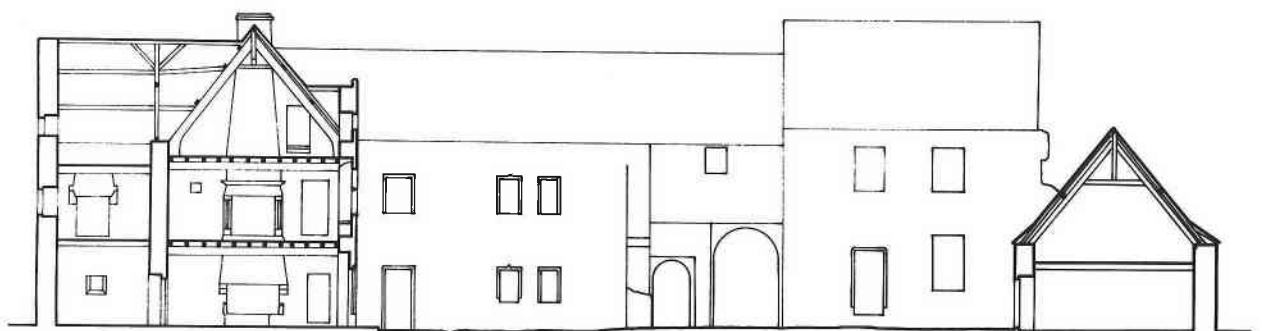
COUPE VV VERS LE NORD
