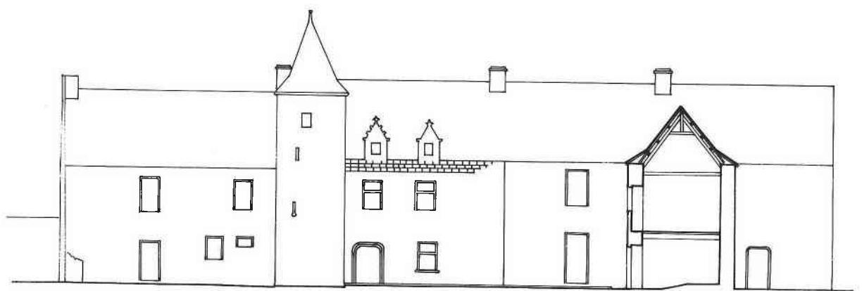
COUPE WW
