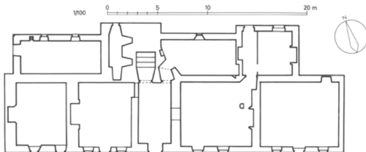
PLAN DU REZ DE CHAUSSEE NIVEAU W W
