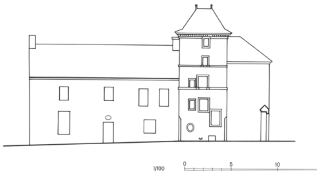
façade sud
