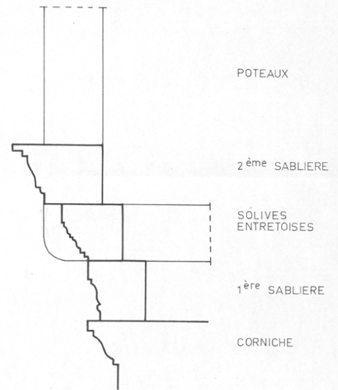
schéma de l'encorbellement du premier étage
