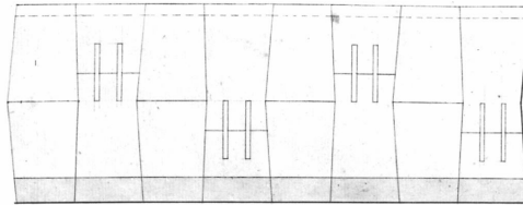
Coupe du Déversoir de Châteaulin. (levée en 1845.)
