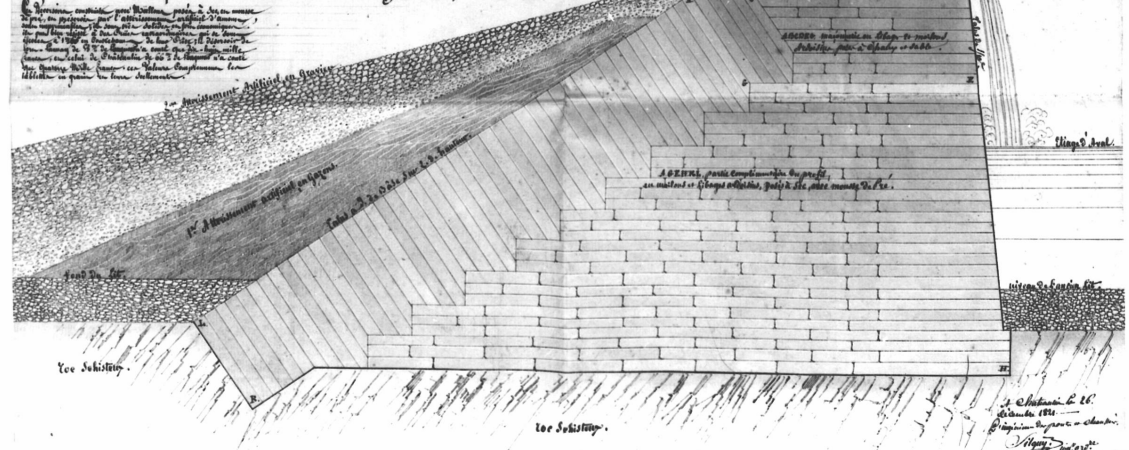
Coupe du Déversoir de Port-Launay. (levée en 1845.)
