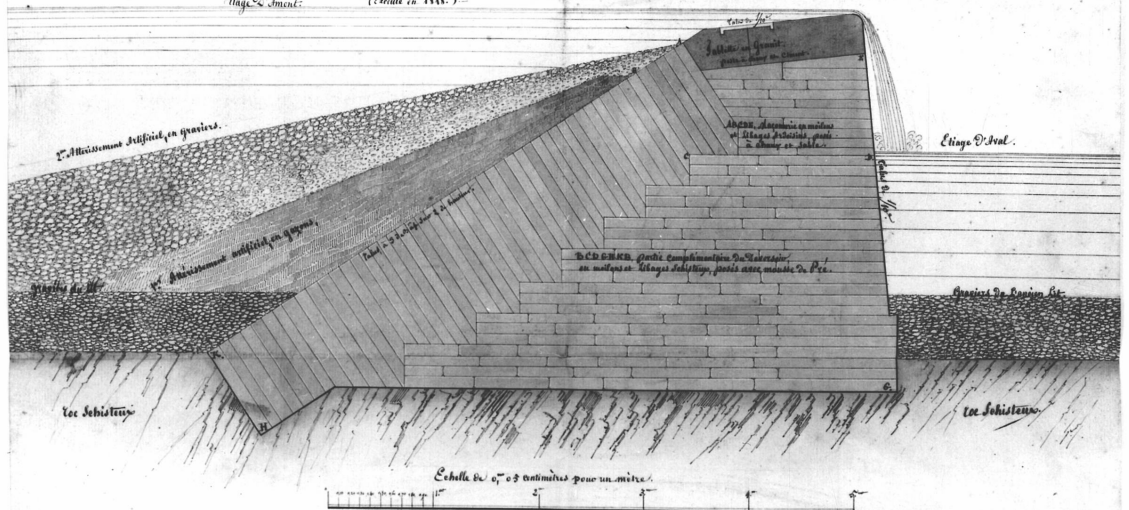
Coupe du Déversoir de Châteaulin. (levée en 1845.)
