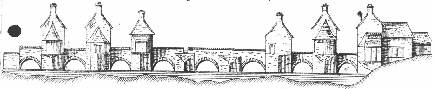
Élévation géométrale du vieux pont de châteaulin.
