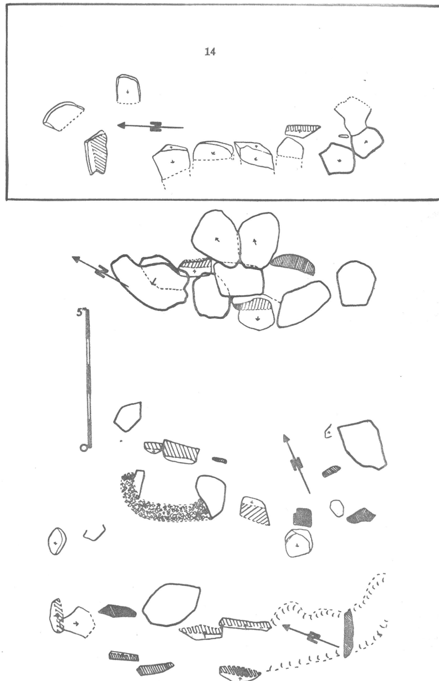
Fig. 5. Sépultures mégalithiques de la Ville-Boscher, Guer ; le Clos-Boscher, Monteneuf ; le Grand-Village (Ouest), Caro et Bramblay, Campénéac.
