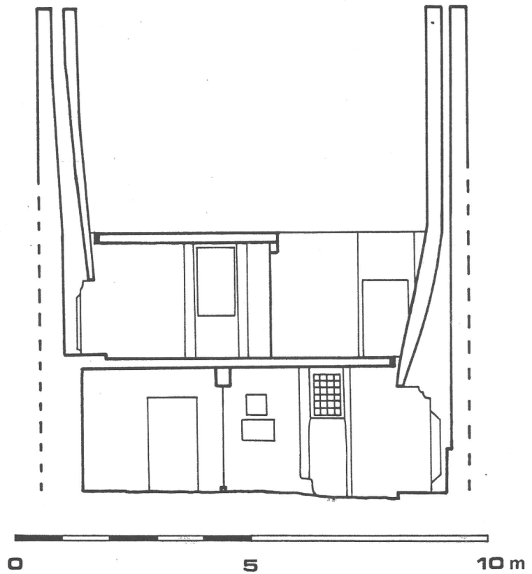
- coupe longitudinale
