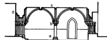
COUPE WW
