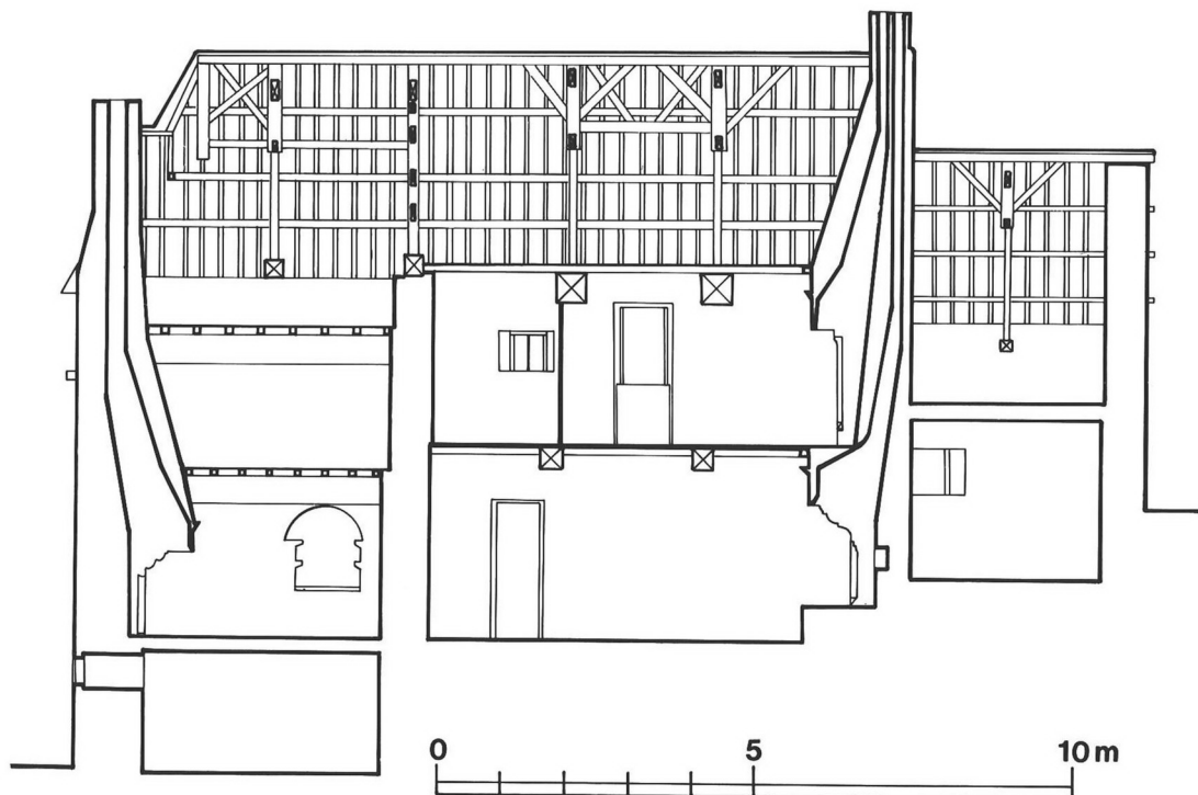
Coupe A-A'
