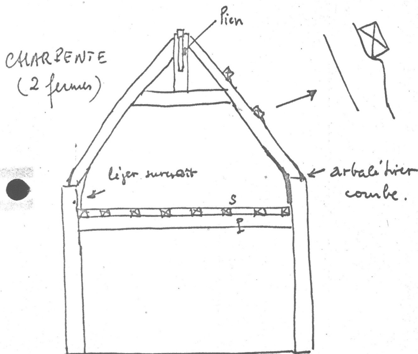
COUPE TRANSVERSALE
