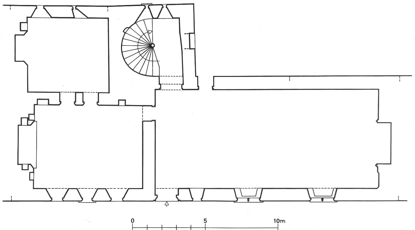
Plan au sol
