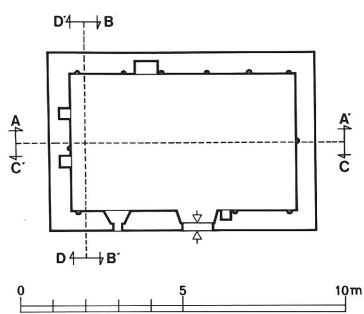
Plan au sol
