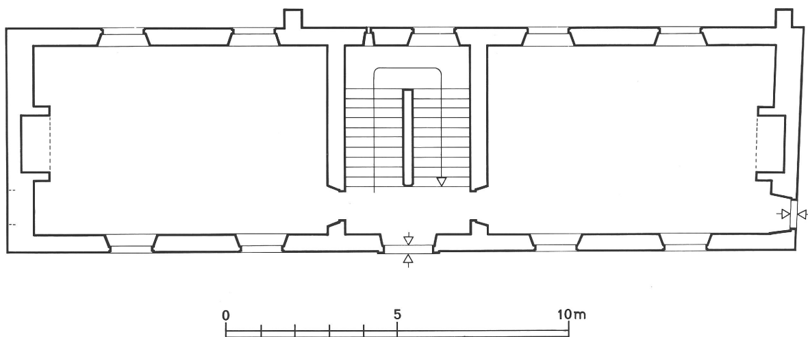
Plan au sol
